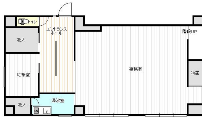
1階 平面図
